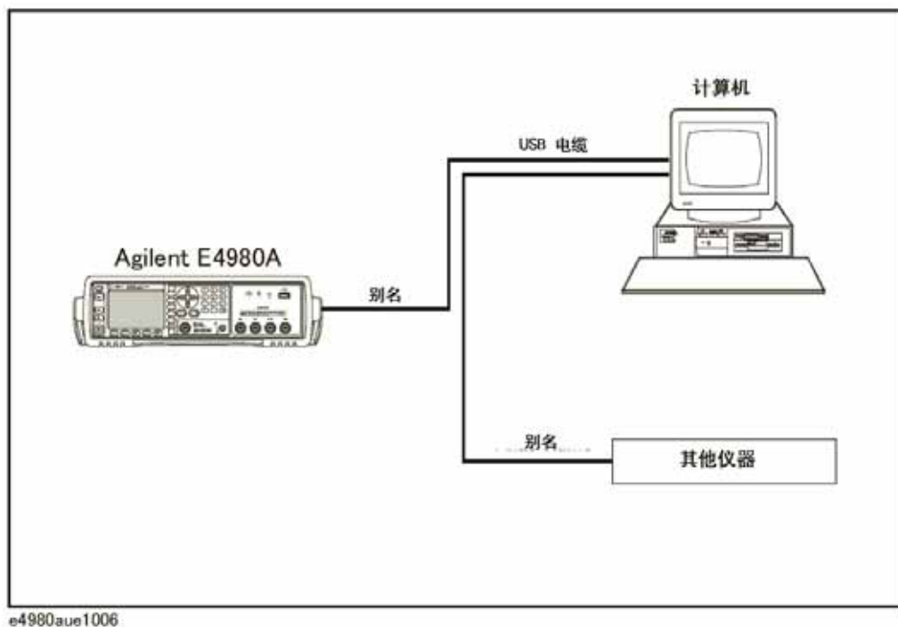
USB远程控制系统的配置
