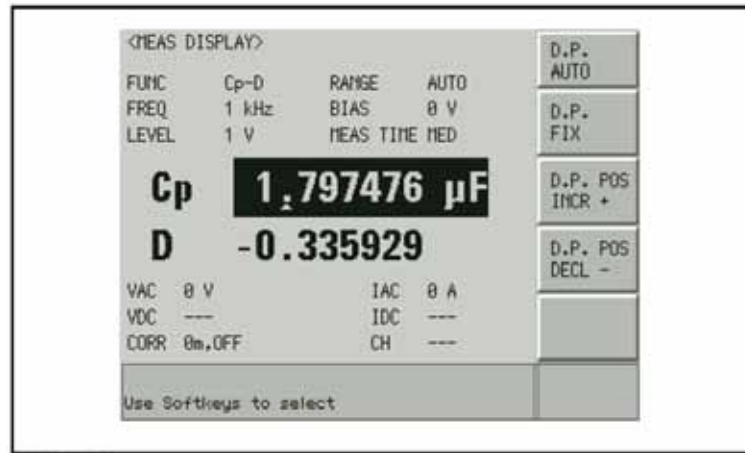
测量结果的固定显示示例
