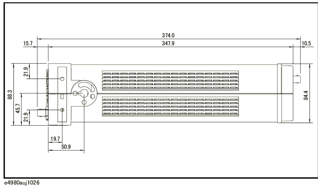
图11-7 尺寸（侧视图，不带把手和减震垫，单位毫米，额定值）
