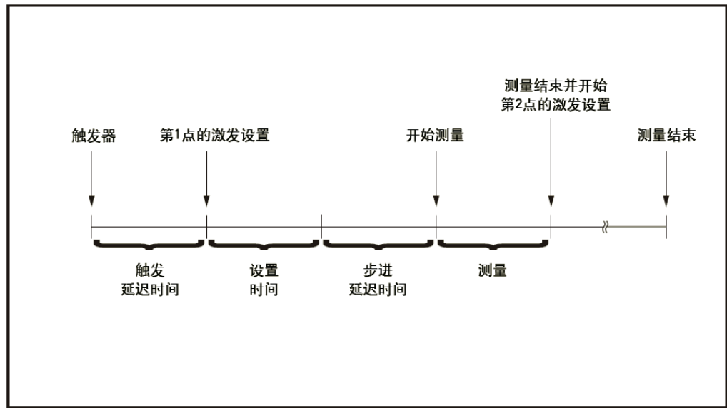
图4-5 触发延迟时间和步进延迟时间
