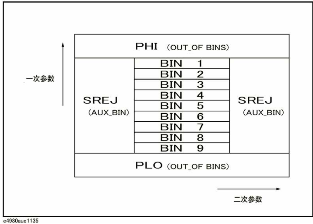
/PHI、/PLO和/SREJ信号区域的示例（比较器）
