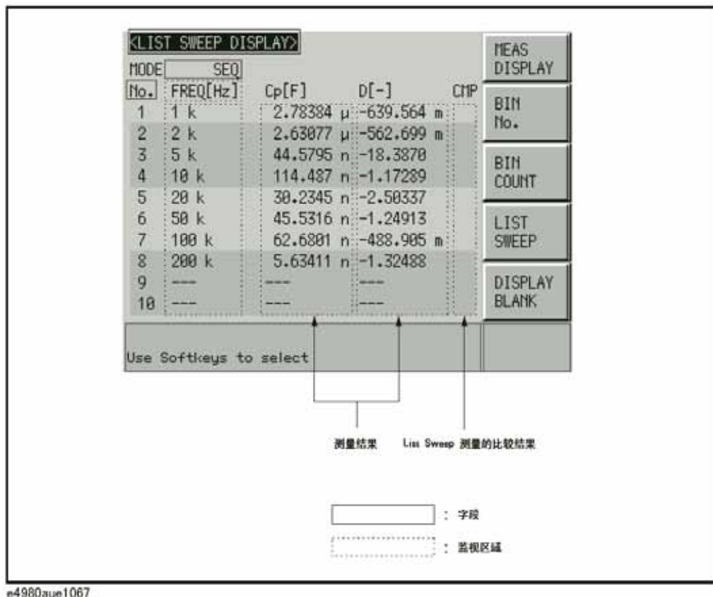
LIST SWEEP DISPLAY页面
