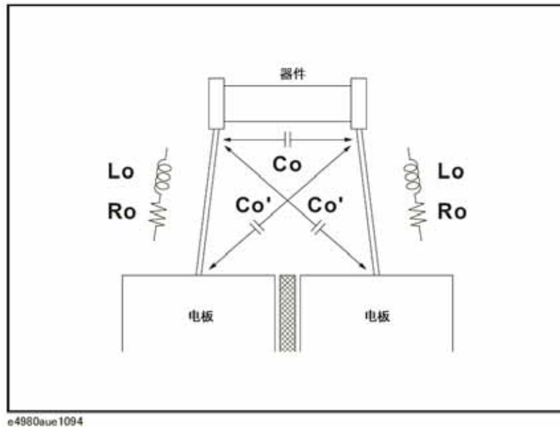
寄生阻抗模型（使用Keysight16047A/D/E）
