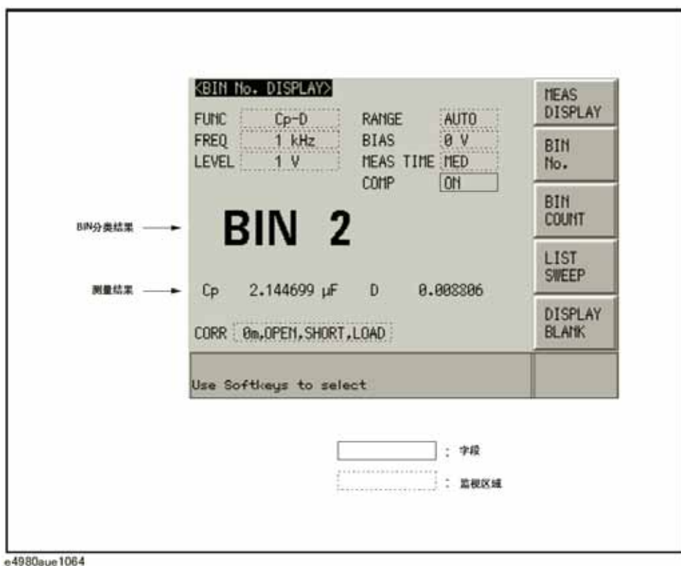
图3-9 BIN NO. DISPLAY页面
