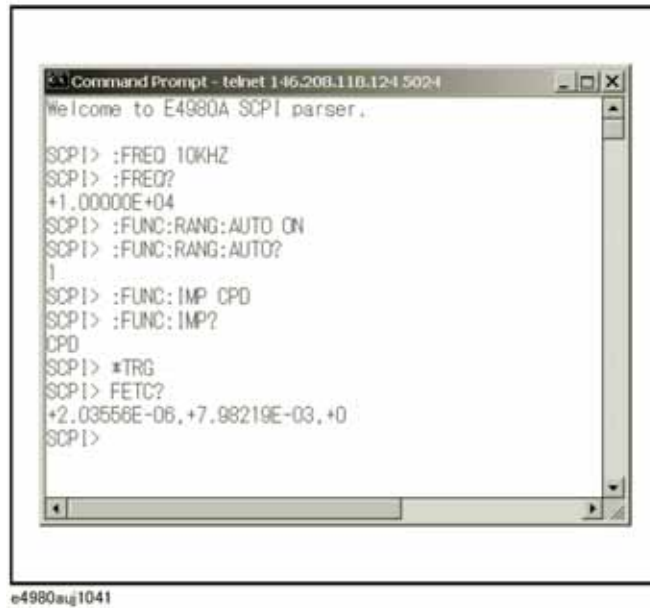
图 8-4 使用telnet的控制示例
