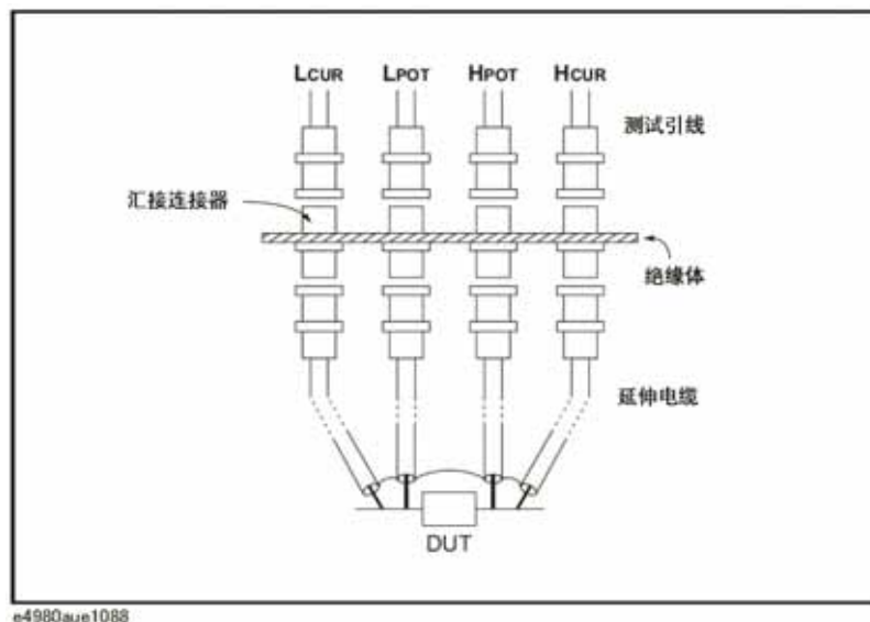
延伸四端对测试引线
