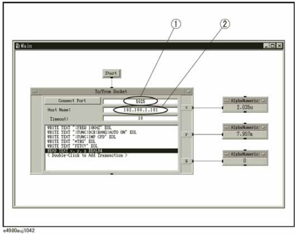
图 8-5 使用Keysight VEE的控制示例
