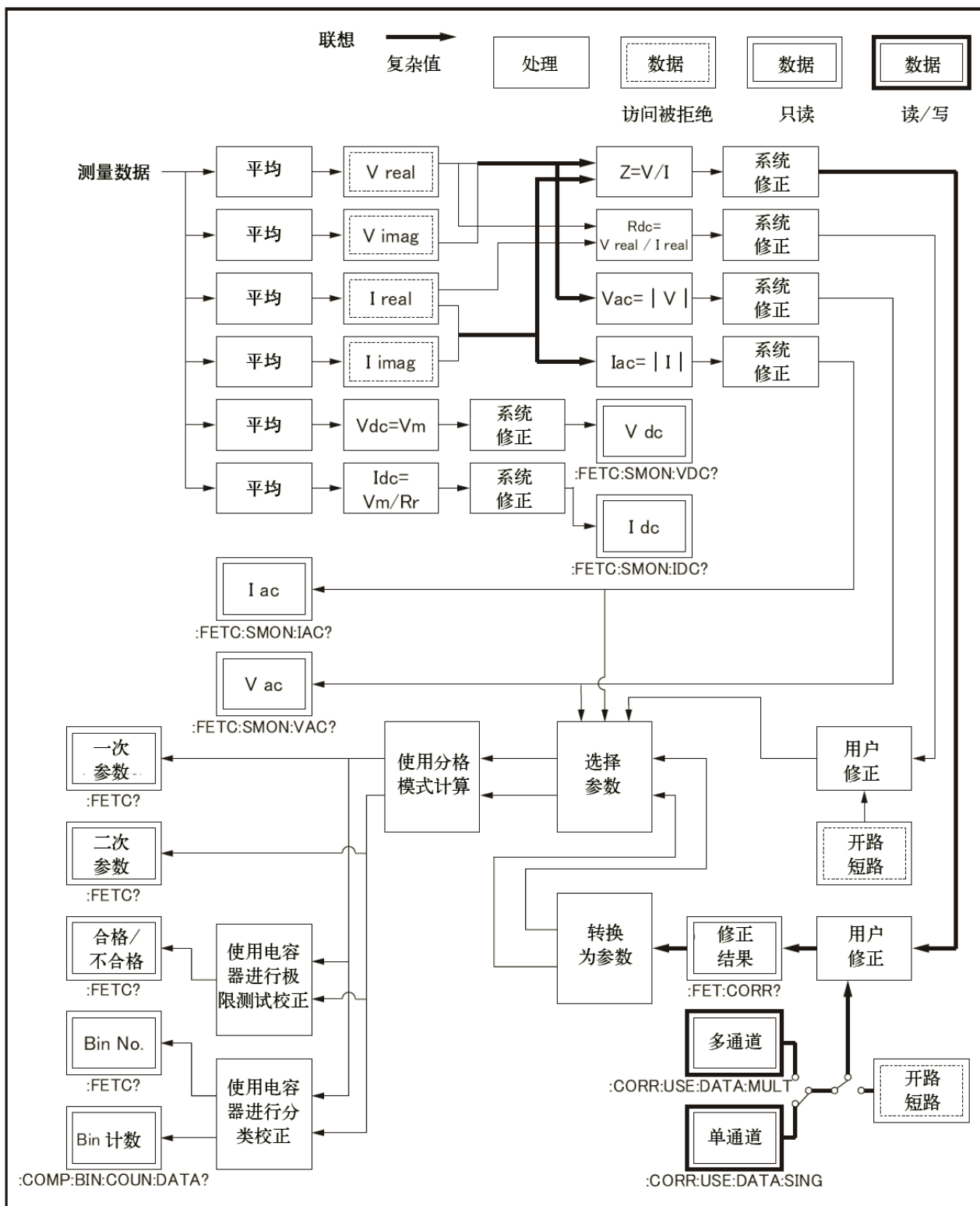
图10-1 数据处理流程图
