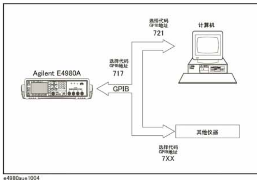
GPIB远程控制系统的配置
