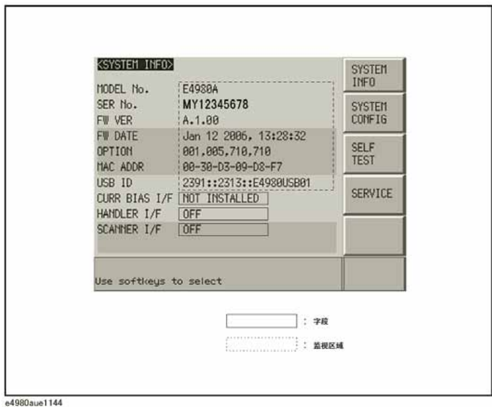
图5-1 SYSTEM INFO页面
