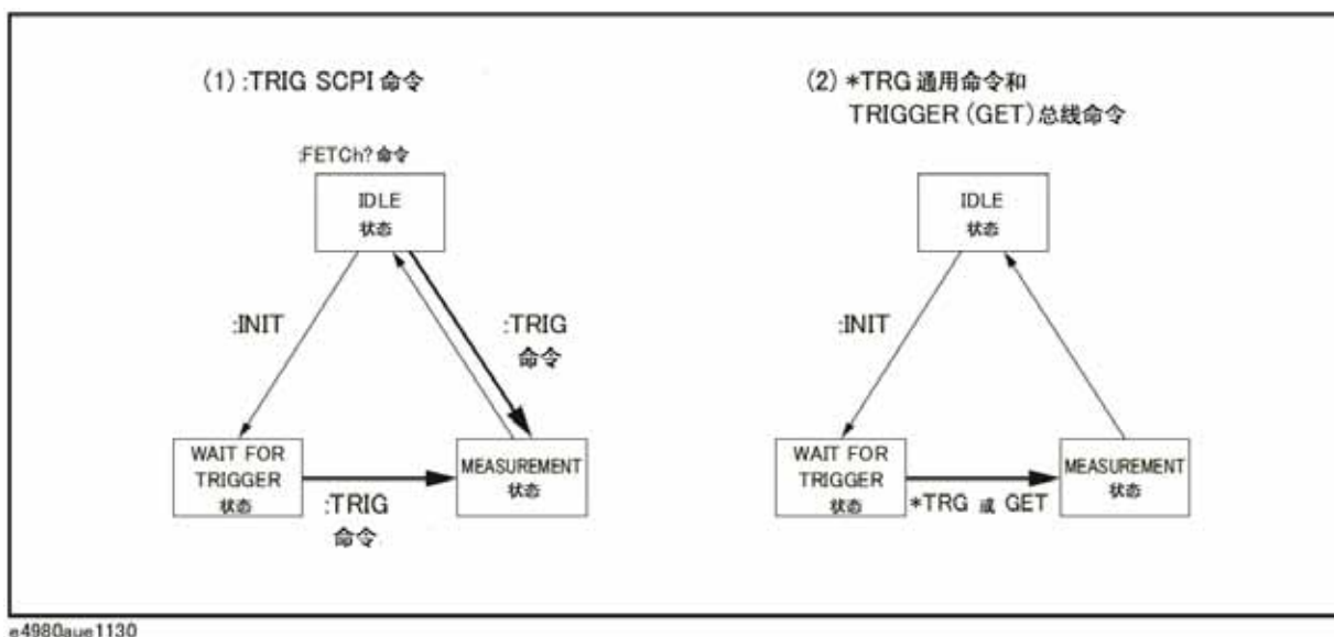
图8-14 触发系统和触发命令
