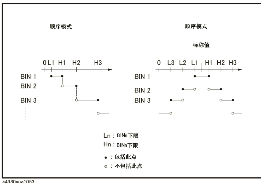
图4-16 容限模式和顺序模式
