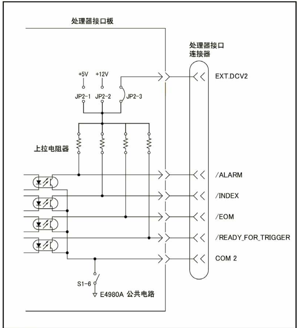
图E-7 控制输出信号的输出电路配置
