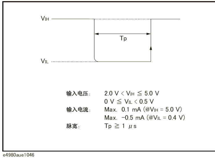
图4-2 外触发脉冲
