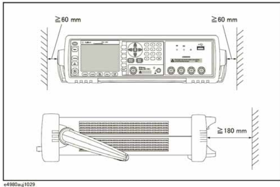
安装的通风间隔
