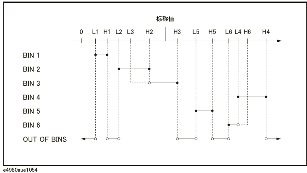
容限模式中的分类示例
