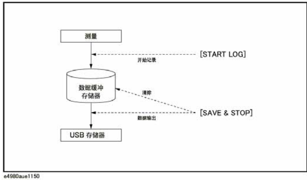
图6-5 将测量结果保存到USB存储器
