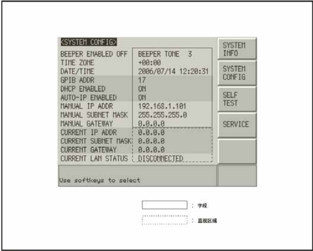
SYSTEM CONFIG页面
