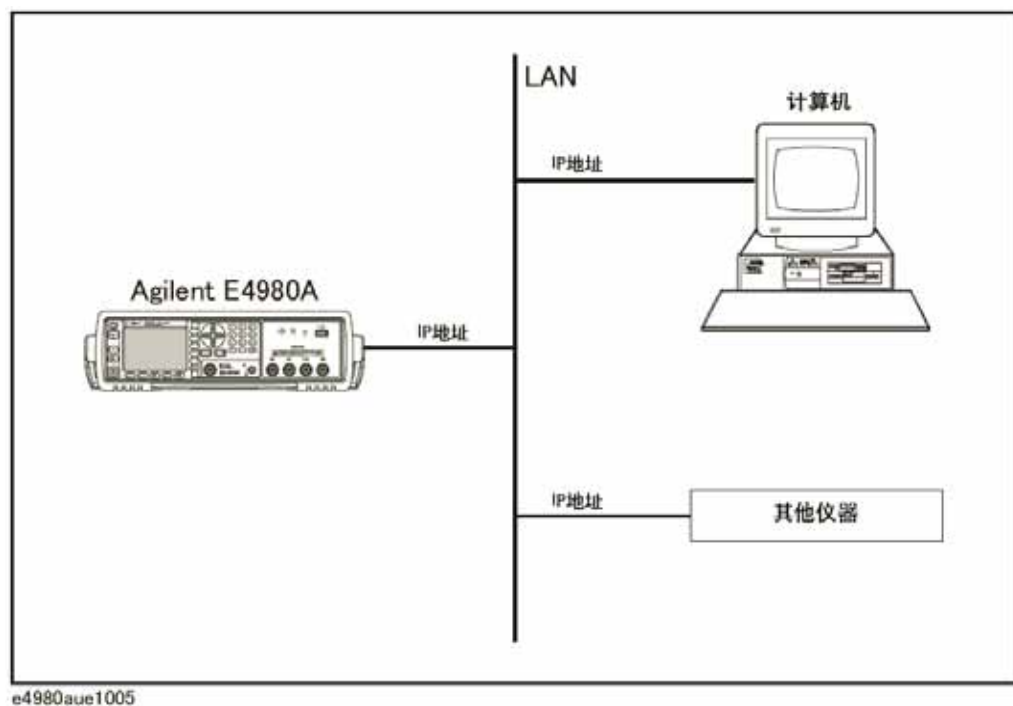
LAN远程控制系统的配置
