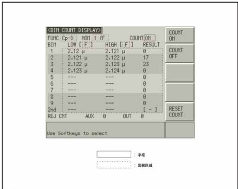
BIN COUNT DISPLAY页面
