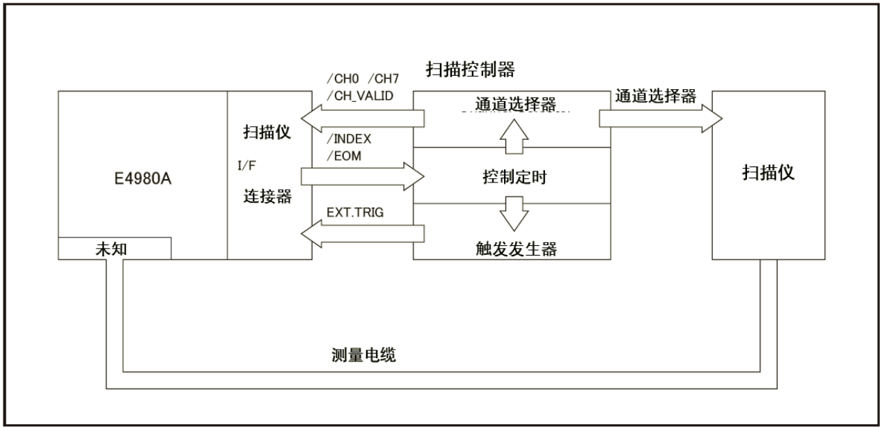
图F-5 对扫描仪接口进行系统配置的示例
