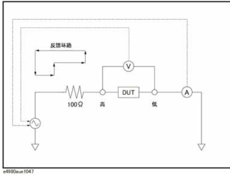
图4-3 反馈电路
