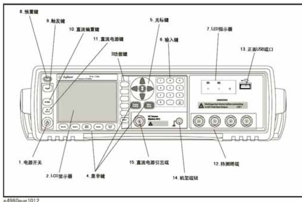
前面板
