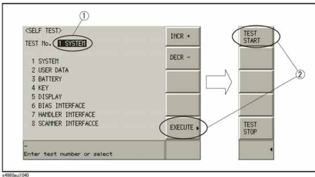
自检屏幕和程序
