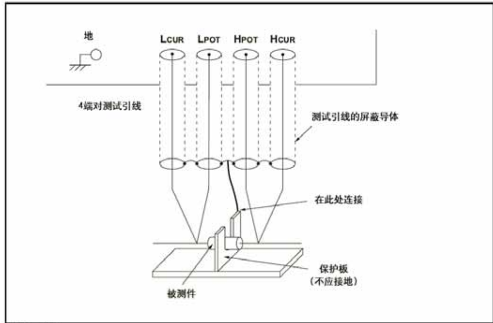
被测件保护板连接示例
