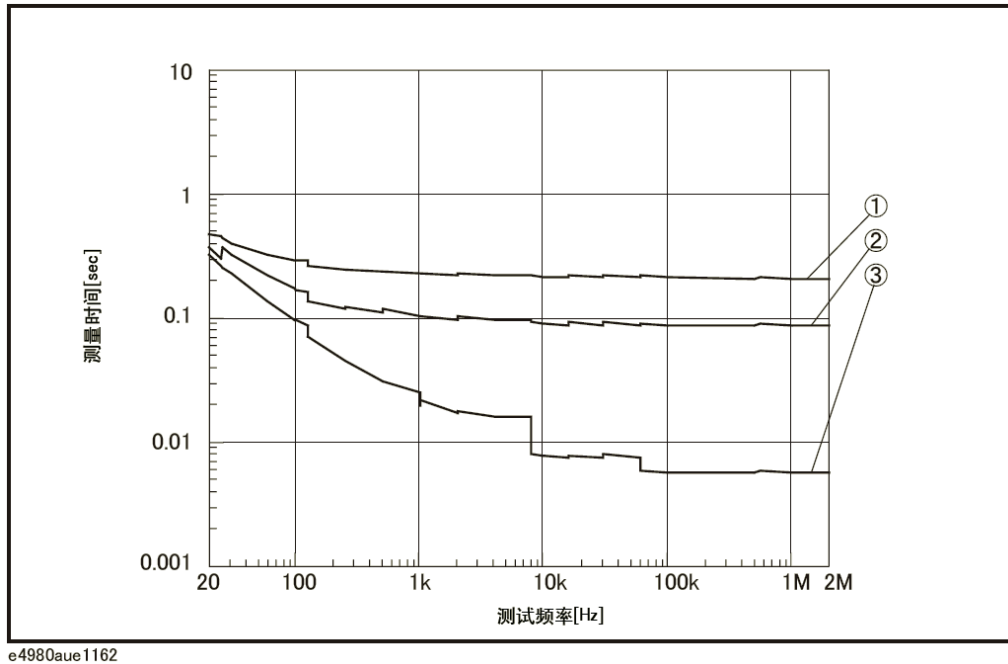
图11-9 测量时间 (直流偏置: 切断)
