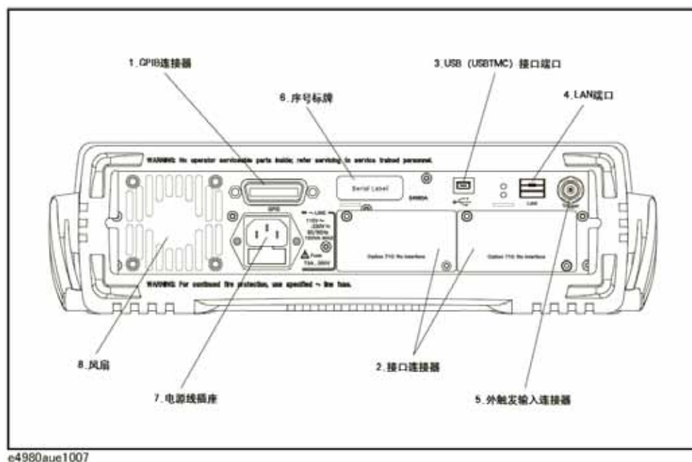
后面板
