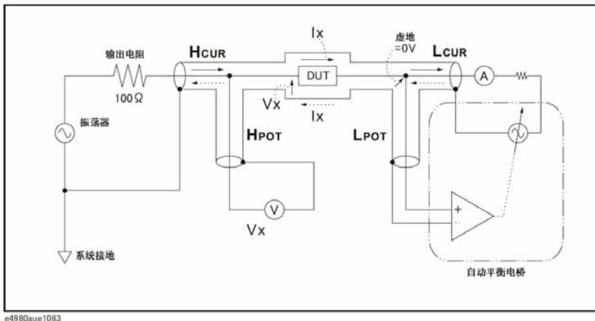
图7-7 四端对测量原理
